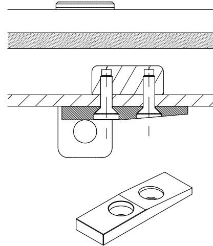
A-A
