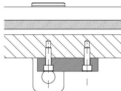
B-B
