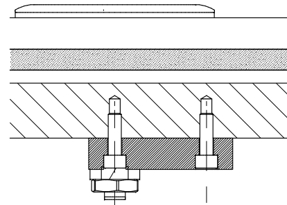
B-B
